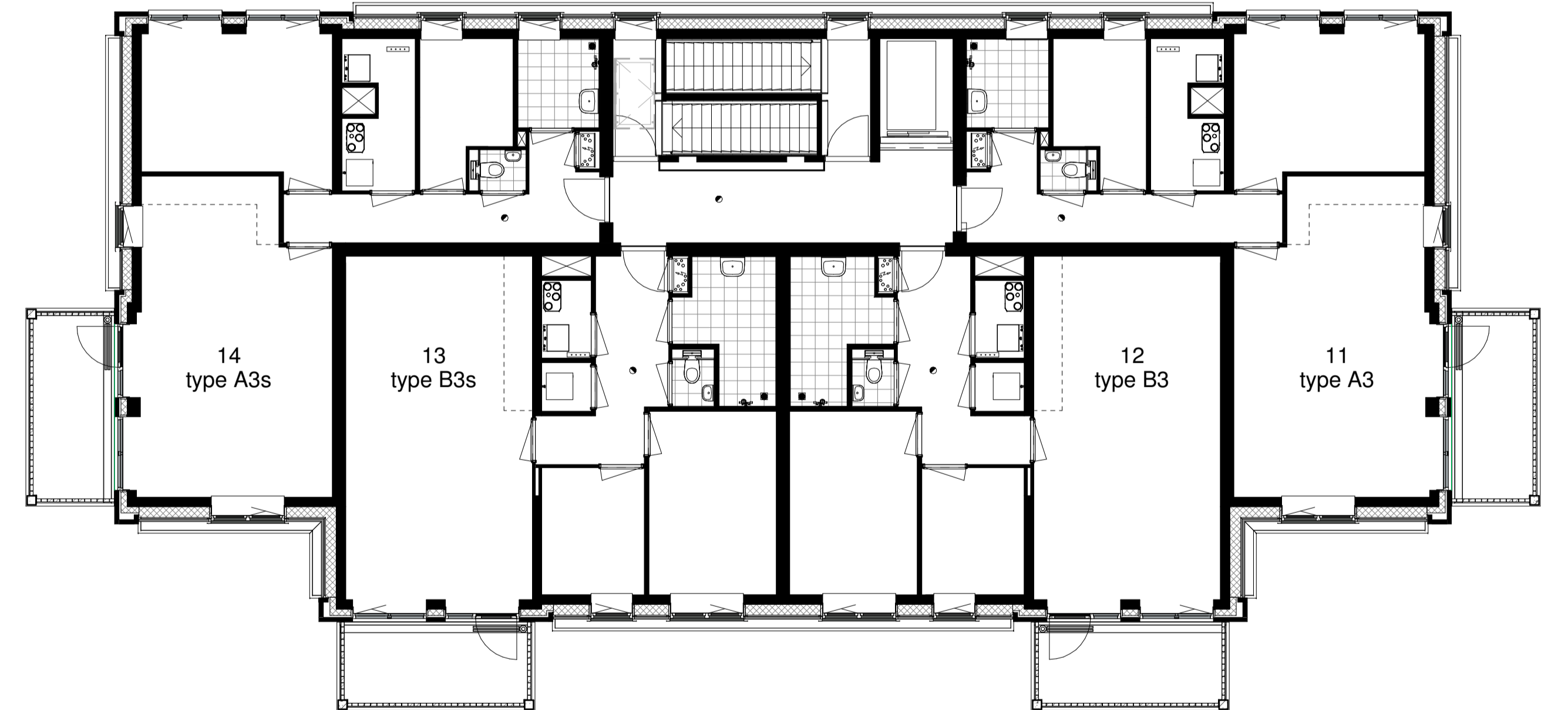
derde verdieping
